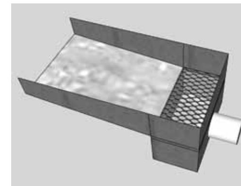
Figura 08 – Esquema da calha com tela para pré-limpeza de impurezas
