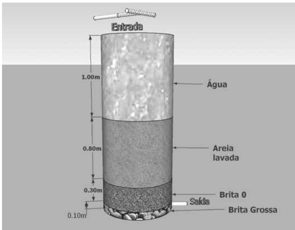
Figura 10 – Esquema do interior do filtro lento
