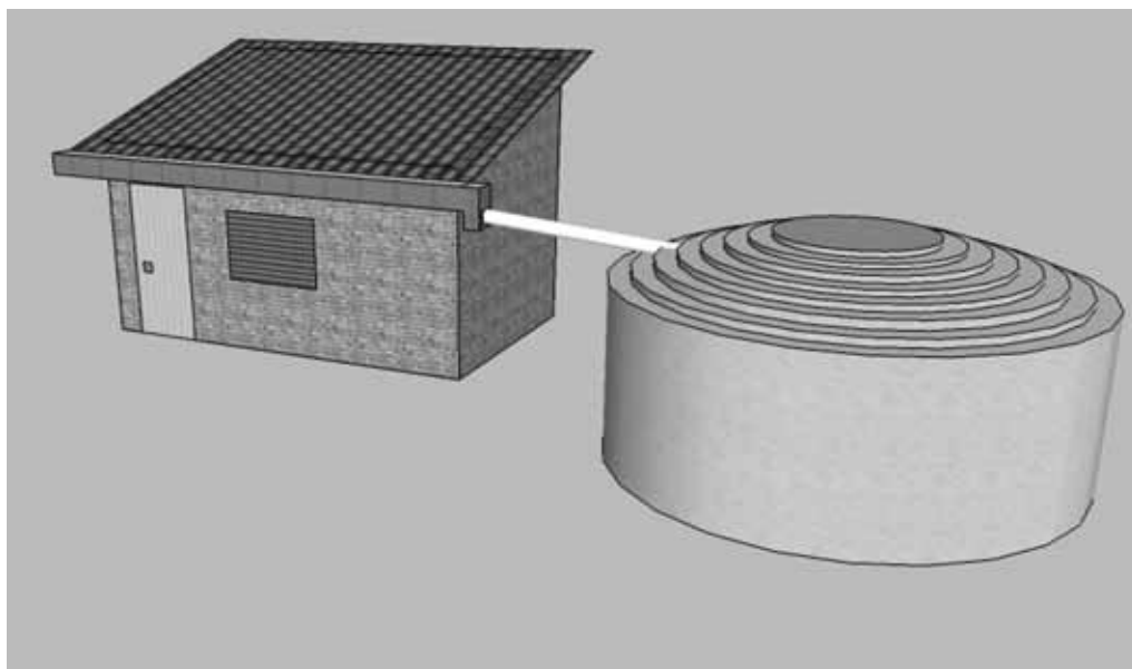
Figura 7 – Esquema de coleta de água de chuva
