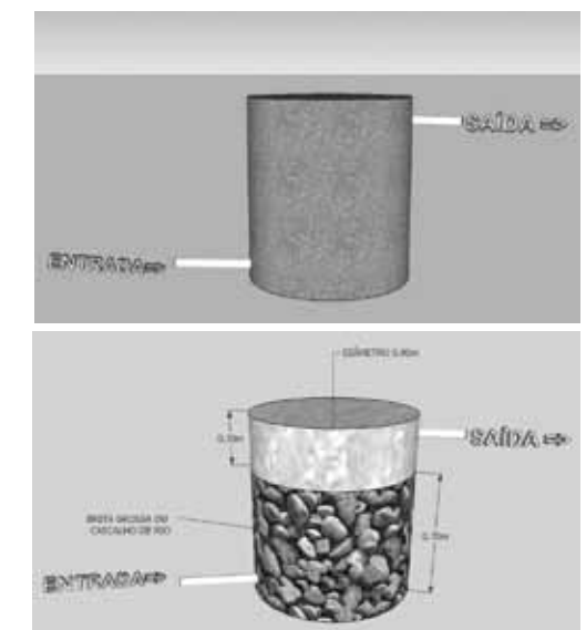
Figura 03 – A) vista externa do pré-filtro B) Vista interna e dimensões
