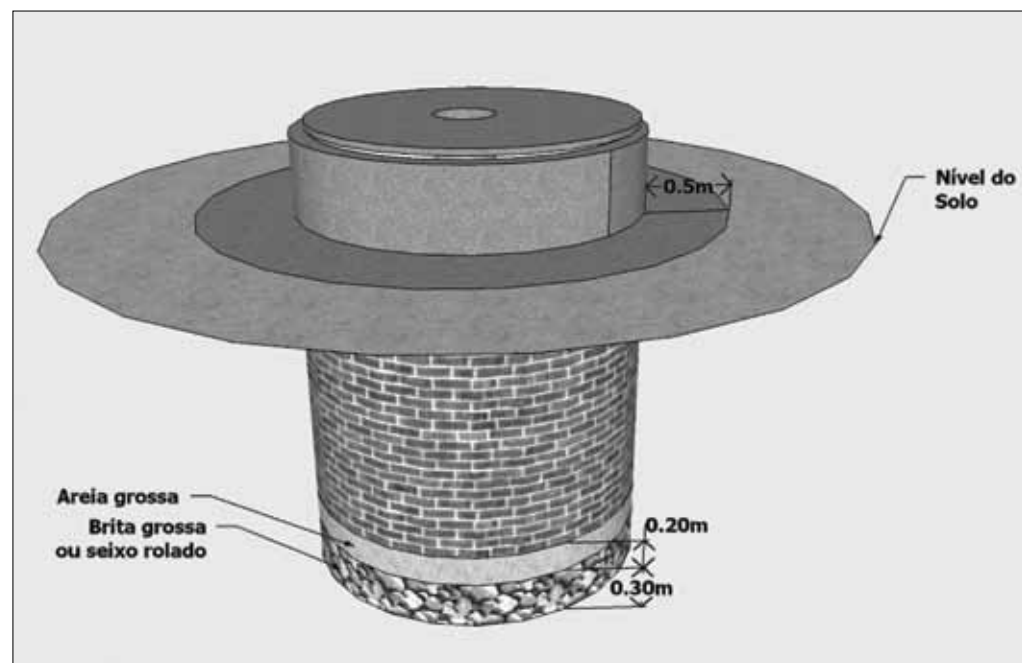
Figura 6 – Esquema geral de construção de cisterna
