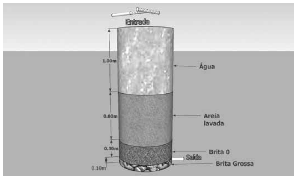
Figura 04 – Vista interna do filtro lento
