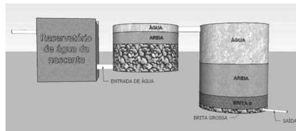
Figura 05 – Esquema geral de filtragem de água de uma nascente
