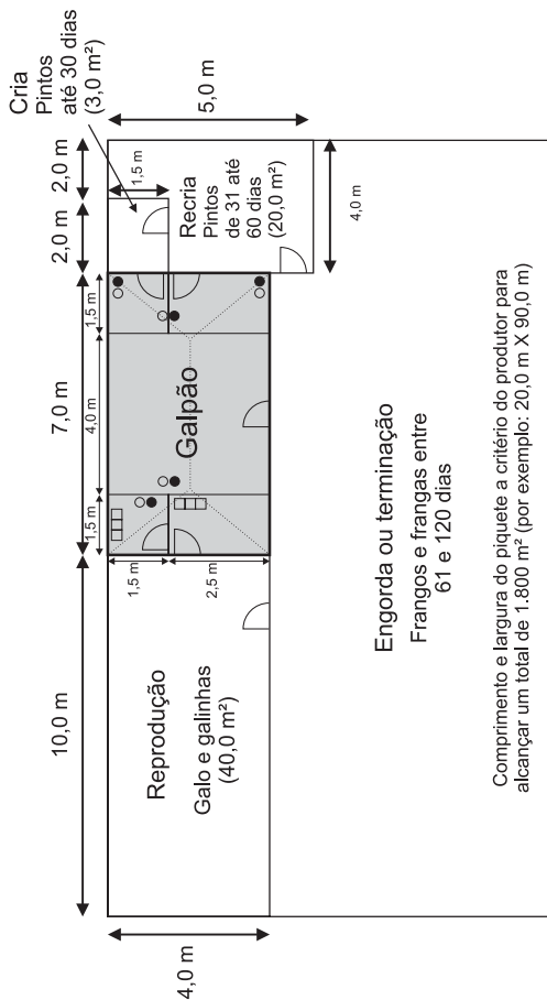
Planta geral com indicação das medidas dos piquetes.
